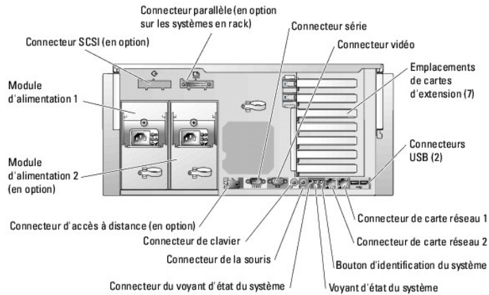
Figure 1-4. Éléments et voyants du panneau arrière
