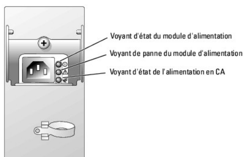
Figure 1-5. Voyants des modules d'alimentation redondants
